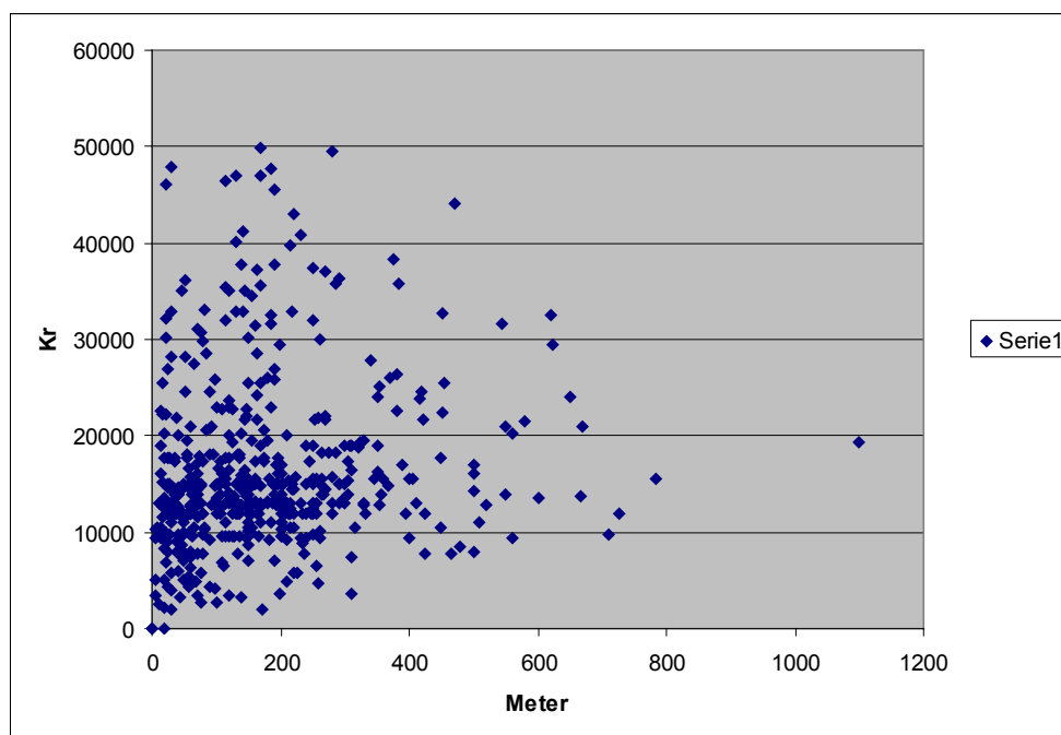
Figur 2: Anslutningskostnad i relation till fågelvägsavstånd till närmaste befintliga transformatorstation (I diagrammet har de tio procent dyraste anslutningarna exkluderats för att få en tydligare bild av fördelningen. Beräkningen av själva genomsnittet görs dock med en statistisk metod som beaktar hela urvalet.
